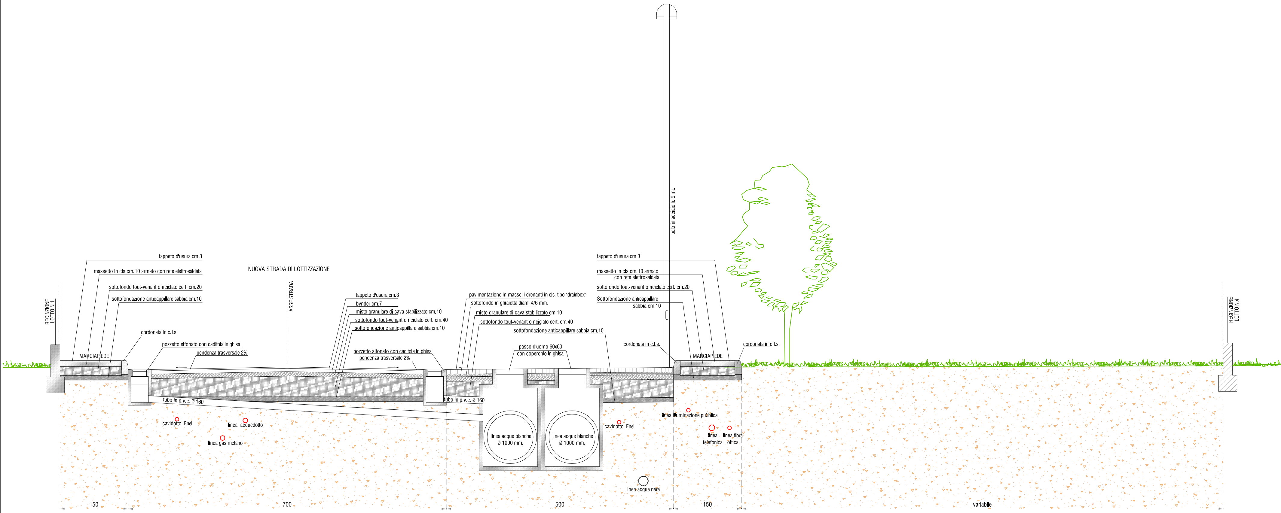
SEZIONE STRADA DI ACCESSO AI LOTTI - scala 1:50
